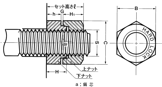
●寸法図
