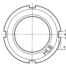
●寸法図
