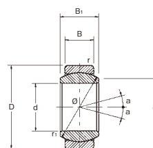
GE・E
