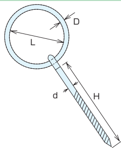
丸カンボルト ROUND RINGS W/BOLT, NUT & WASHER
