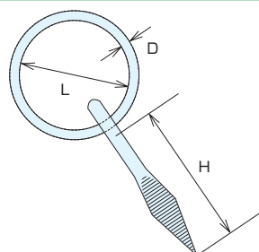
つば付リングボルト RING BOLTS W/SHOULDER
