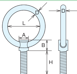
リングナット RING NUTS
