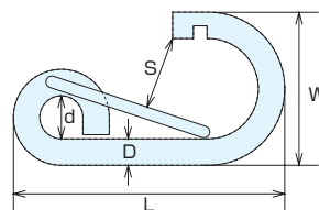
R型フック SPRING SNAPS "R", TYPE
