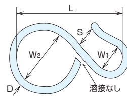
パイプSカン PIPE "S" HOOKS
