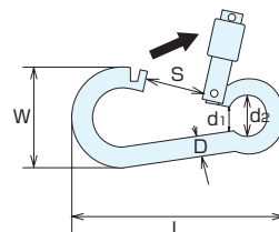
オープンフックB型 OPEN HOOKS
