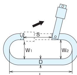
オープンフックP型 "PUCHI-KARABINA" OPEN HOOKS
