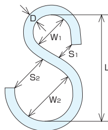
パイプSカン PIPE "S" HOOKS
