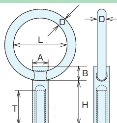
リングナット RING NUTS
