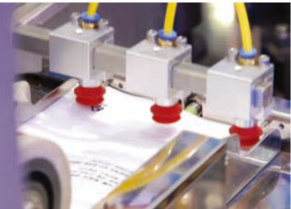
▲ ビニール袋開封
