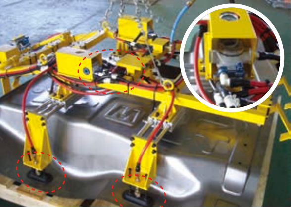
▲ 自動車産業 (各種パネル搬送)
