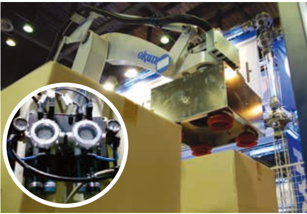
▲ パレタイジングロボットのボックスハンドリング
