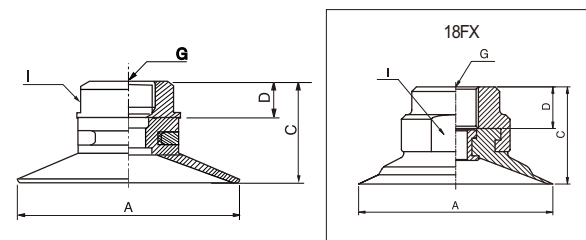
◀ メネジ [mm]
