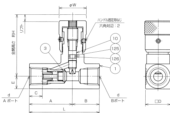
HT-728 (720) -*** スロットルチェックバルブ HT-728 (720) N-*** スロットルバルブ
