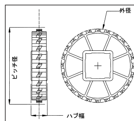
成型スプロケット
