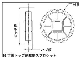
16丁歯トップ側駆動スプロケット
