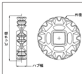
●EZクリーンスプロケット
