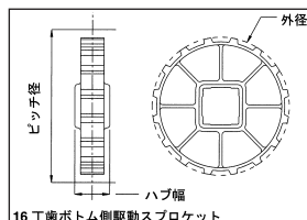
16丁歯ボトム側駆動スプロケット
