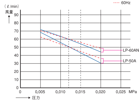
LP-50A・60AN
