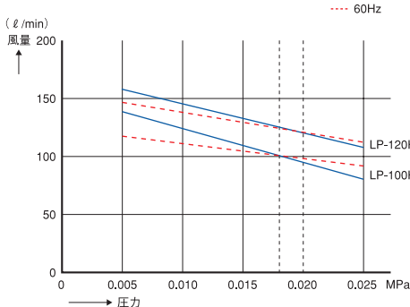
LP-100H・120H
