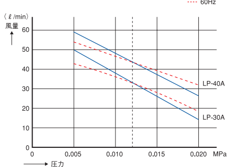
LP-30A・40A
