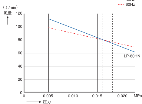
LP-80HN
