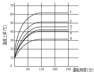
(図2) S6R 06GD (モーター単体)
