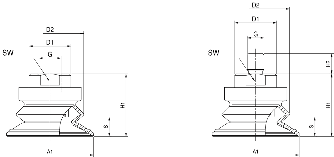
▲ VBF 25PU、VBF 30PU、VBF 40PU、VBF 50PU
